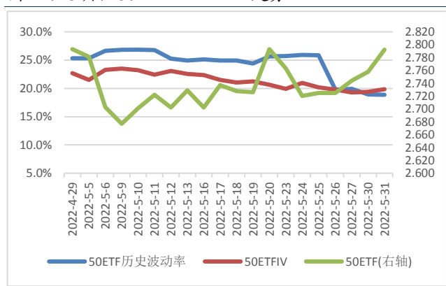
图 24：5 月，50ETF、HV、IV 走势
